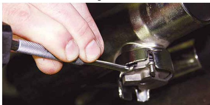
4. Montage der SMS-Klemme (nur leicht schlagen, da ansonsten die Klemme verformt werden könnte und somit Ihre Fixierung verliert)
